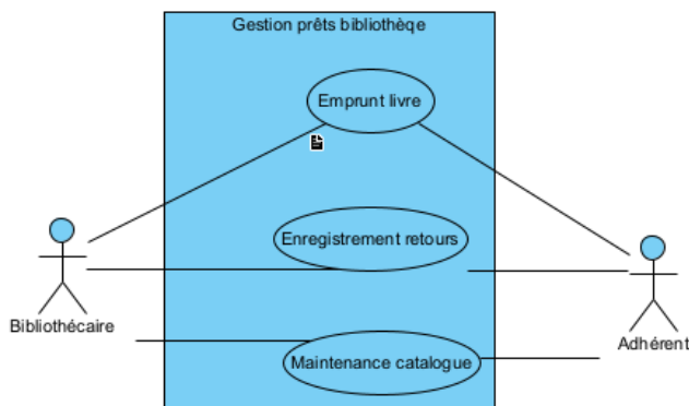
Figure 1 : Diagramme de cas d'utilisation.
